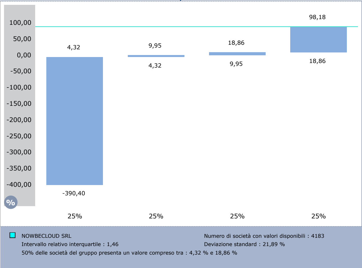
Distribuzione di una variabile: EBITDA/Vendite (%) Ultimo anno disp. - 4183 società
